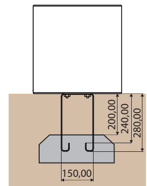
Anclaje a suelos no compactos
