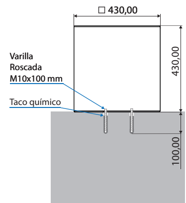
Anclaje a suelos compactos 4 varillas
